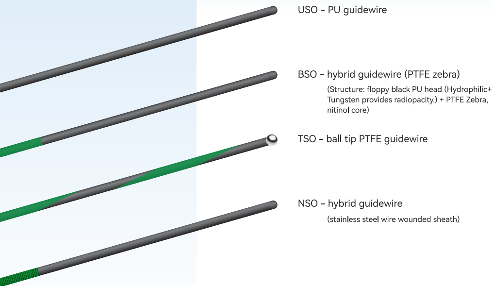
USO - PU guidewire
